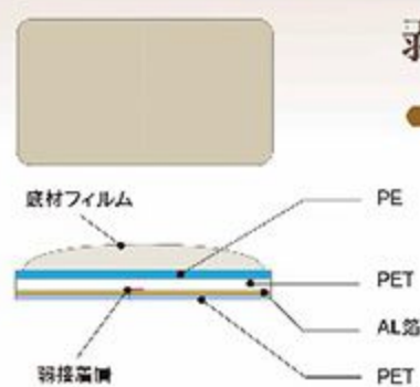
Vパック・ピーリングの断面図
