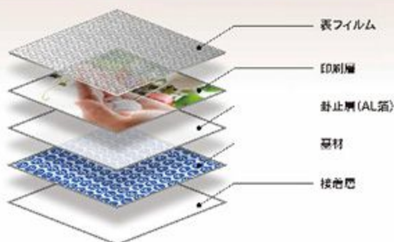
Vパック・ピーリングの上蓋素材構成
